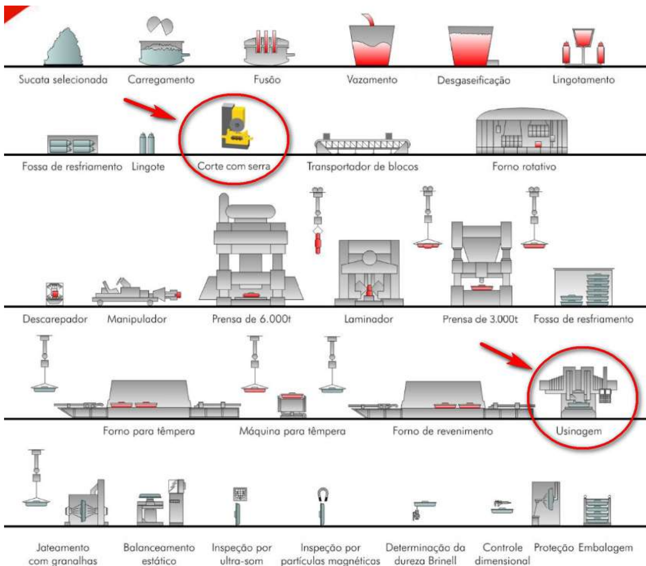
Figura 1 – Desenho esquemático ilustrando o processo da fabricação de rodas ferroviárias.
