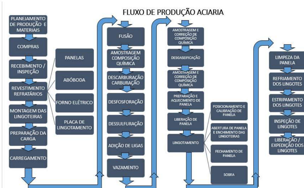
Figura 2 – Fluxo de produção da Aciaria.
