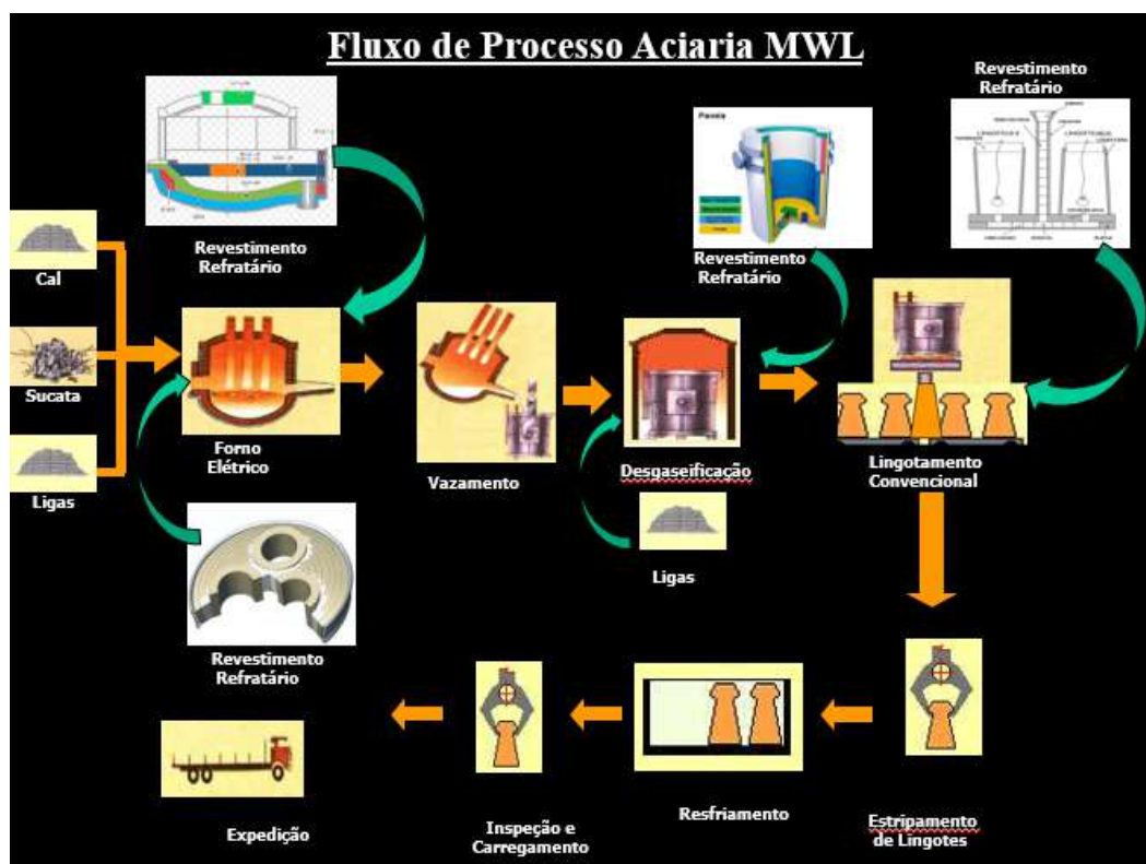
Figura 3 – Fluxo de processos Aciaria
